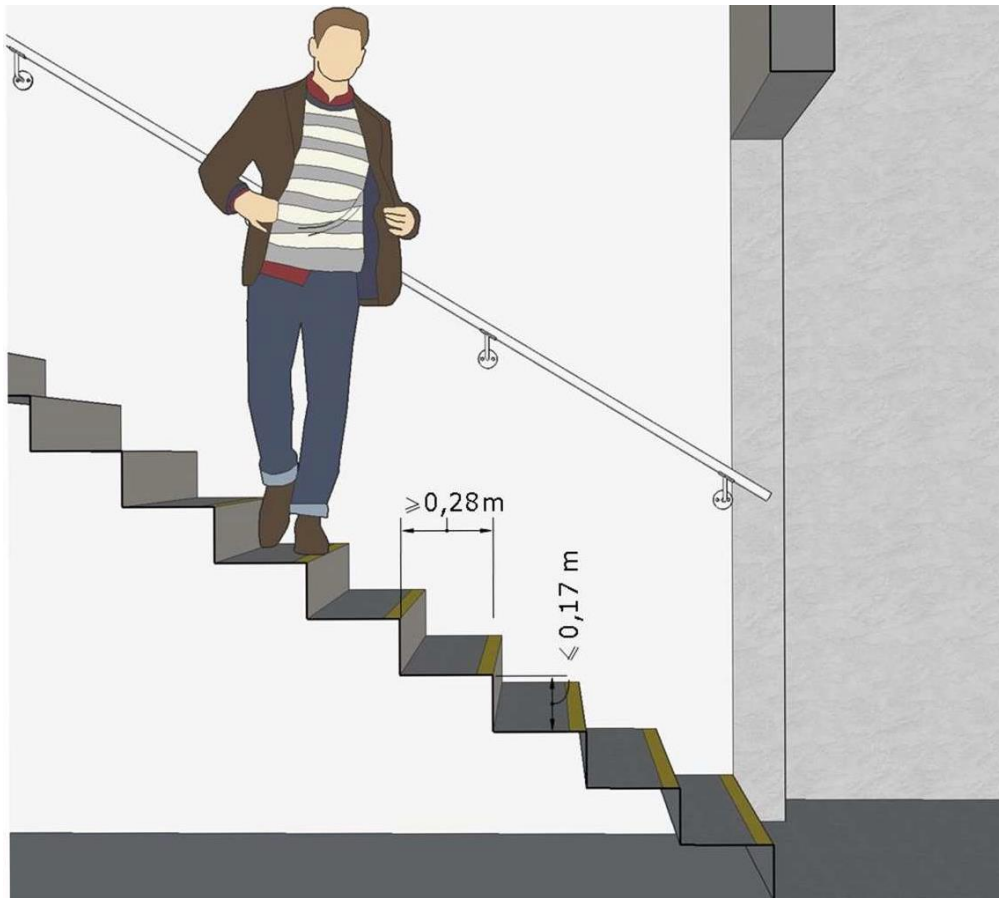
Figure 28.3 Autres configurations d'escaliers rectangulaires (à titre d'exemples)
