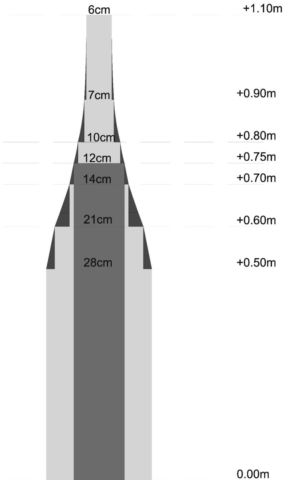
Figure 13.3 Abaque de détection
