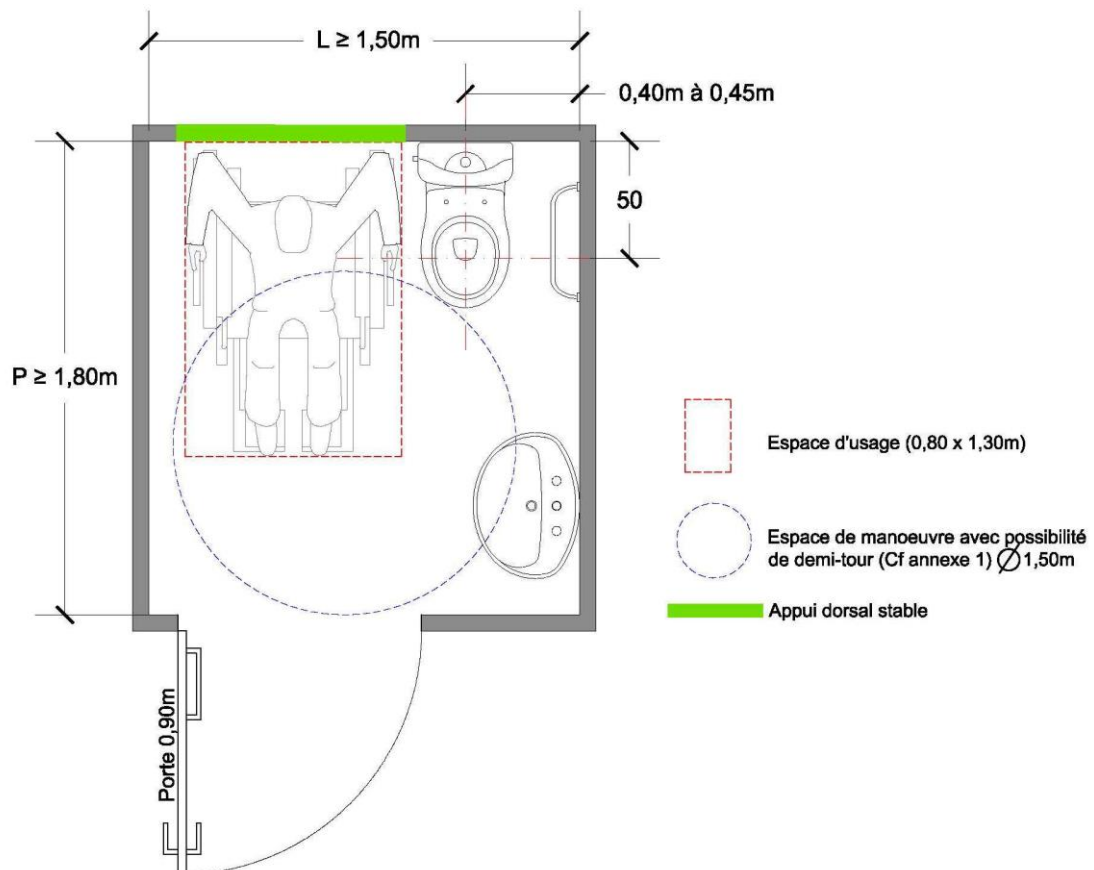
Figure 49.2 Caractéristiques
