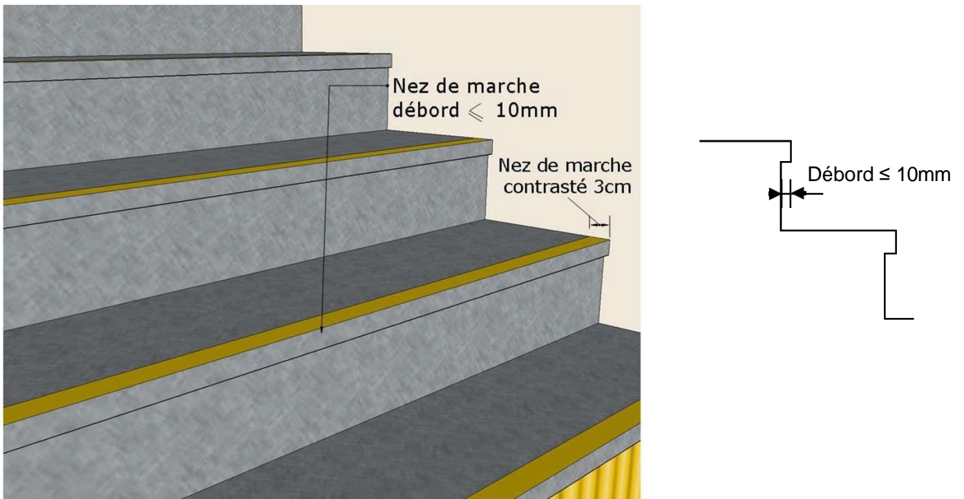
Figure 29.3 Détail nez de marches
