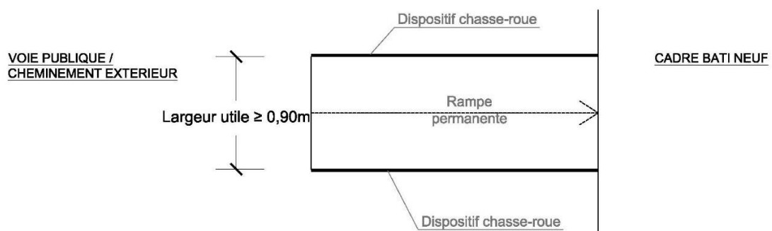
Figure 8.2 – Vue en plan
