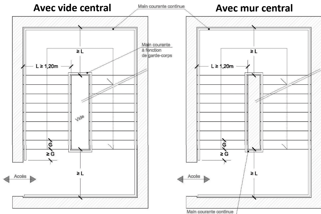
Figure 28.3 Autres configurations d'escaliers rectangulaires (à titre d'exemples)
